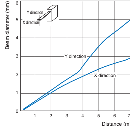
E3C-LR11N
