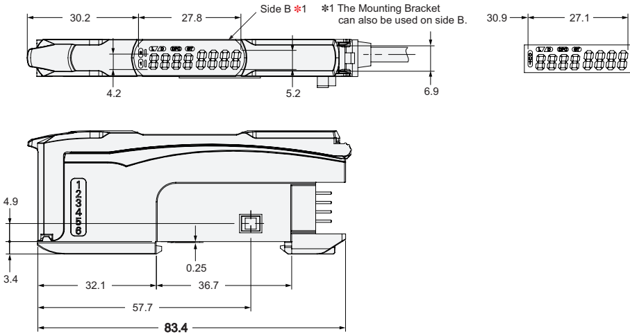
E3C-LDA6N/LDA8N
